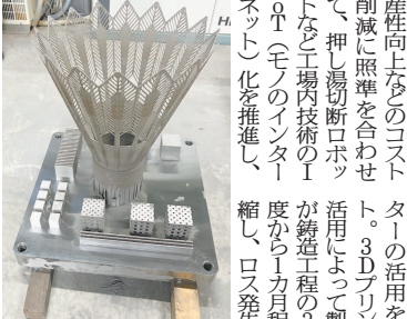
「BLT-S450」で造形したバドミントン羽根
